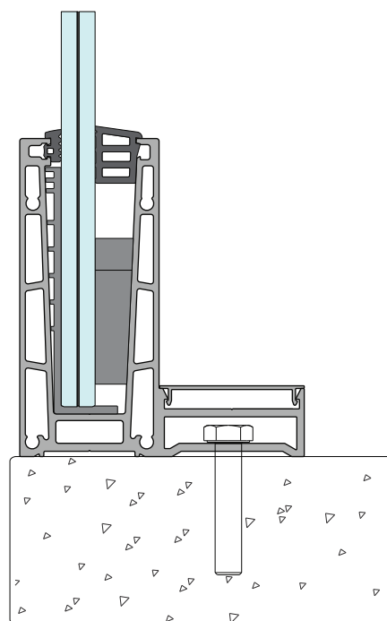
À FACE DA LAGE
