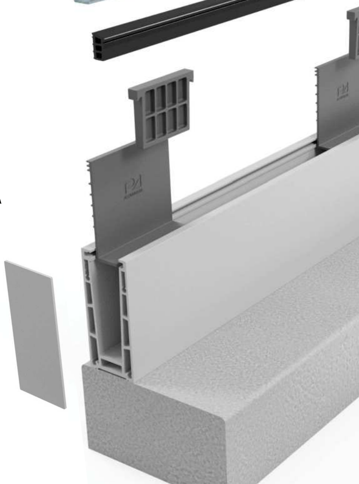
MONTAGEM DA GUARDA
