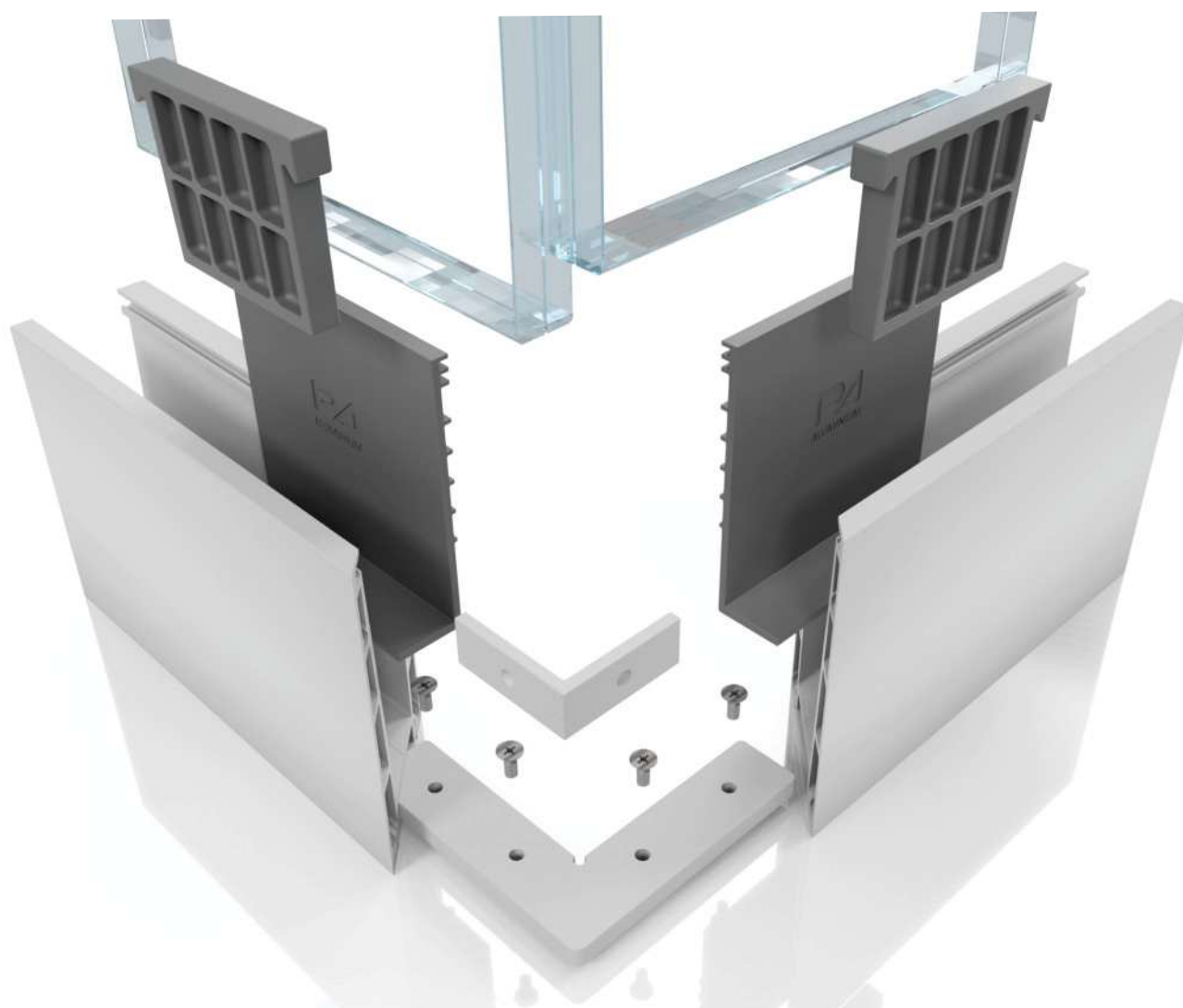
MONTAGEM DO CANTO
