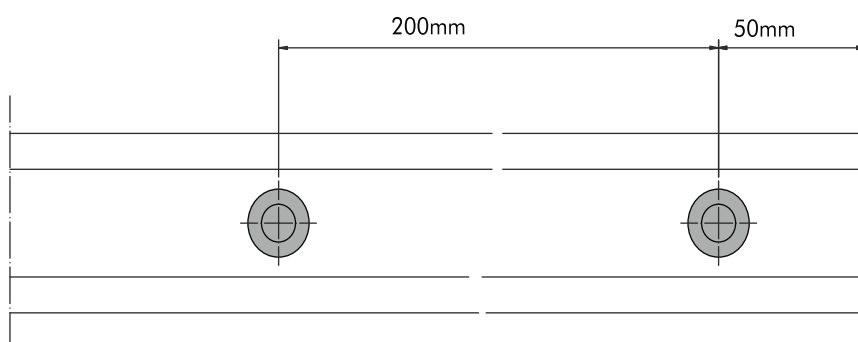
MECANIZAÇÕES SOBRE A LAGE
