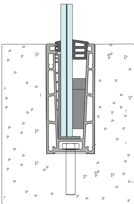
EMBUTIDA NA LAGE
