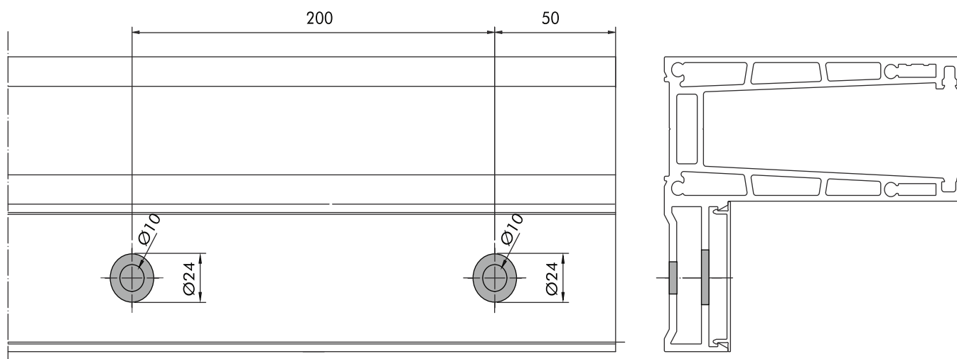
MECANIZAÇÕES À FACE DA LAGE
