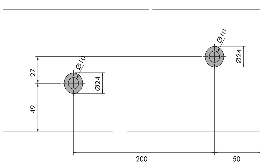
MECANIZAÇÕES À TESTA DA LAGE
